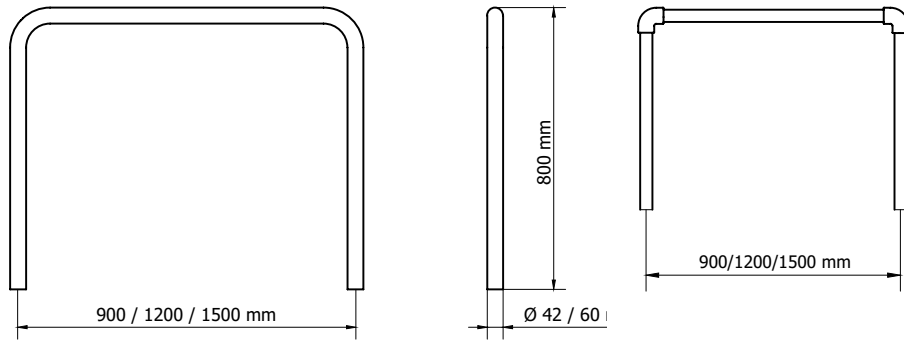
Aanleunrek
